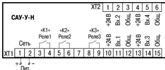
Рисунок 5.1 – Клеммник CAU-Y-N
