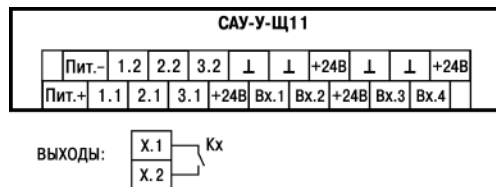
Рисунок 5.2 – Клеммник CAU-Y-Щ11
